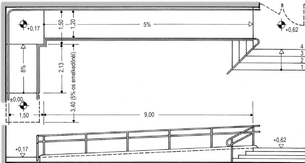
C8. ÁBRA: "L"-ALAKÚ LEJTŐ MEGLÉVŐ LÉPCSŐHÖZ ILLESZTVE
