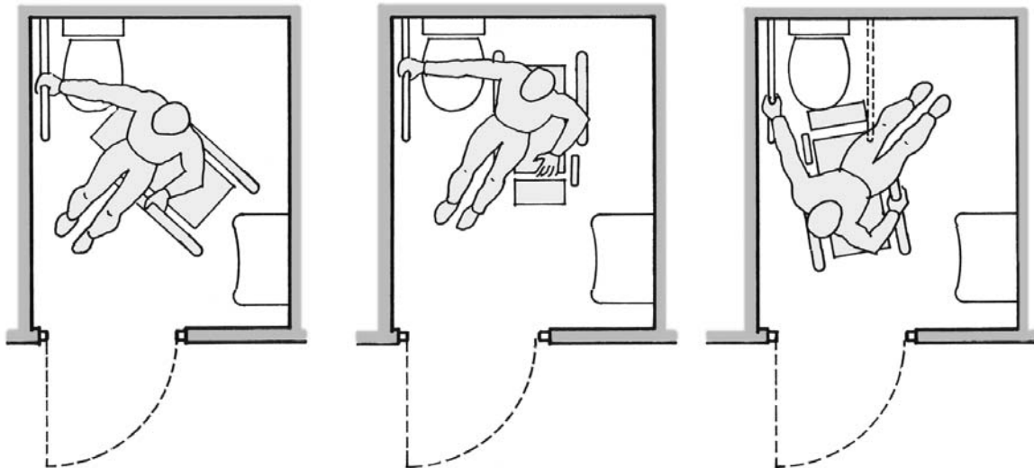
C16. ÁBRA: AZ AKADÁLYMENTES WC-MOSDÓ HELYSÉGBEN A WC-BERENDEZÉS KERÉKESZÉKBŐL VALÓ MEGKÖZELÍTÉSÉNEK LEHETŐSÉGEI
