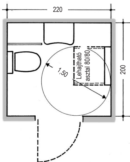
C22. ÁBRA: WC-BLOKK SZÚKÖSEN ÉS ELFOGADHATÓAN MÉRETEZVE
